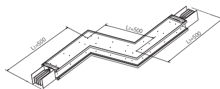
Поперечный Z-модуль
