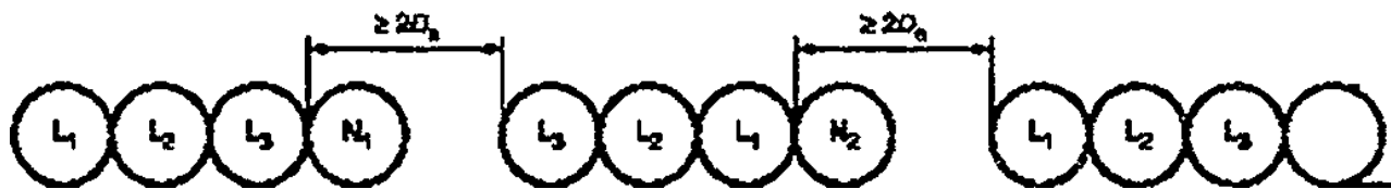
Рисунок Н.52.4 — Специальная конфигурация для девяти параллельных одножильных кабелей в горизонтальной плоскости (см. 523.7)
