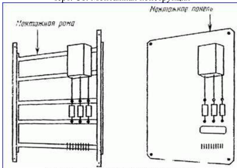
Черт. С9. Неподвижные части
