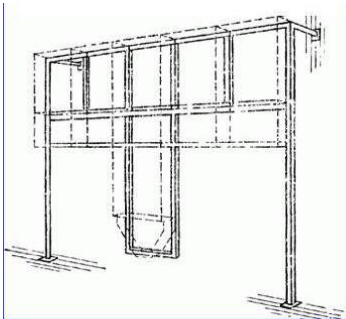
Черт. С8. Монтажная конструкция
