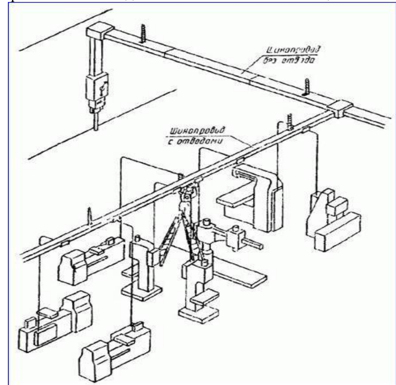
Черт. С7. Система сборных шин (шинопровод)
