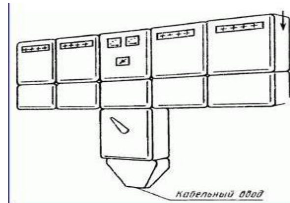
Черт. С6. НКУ заводского изготовления многоящичного типа
