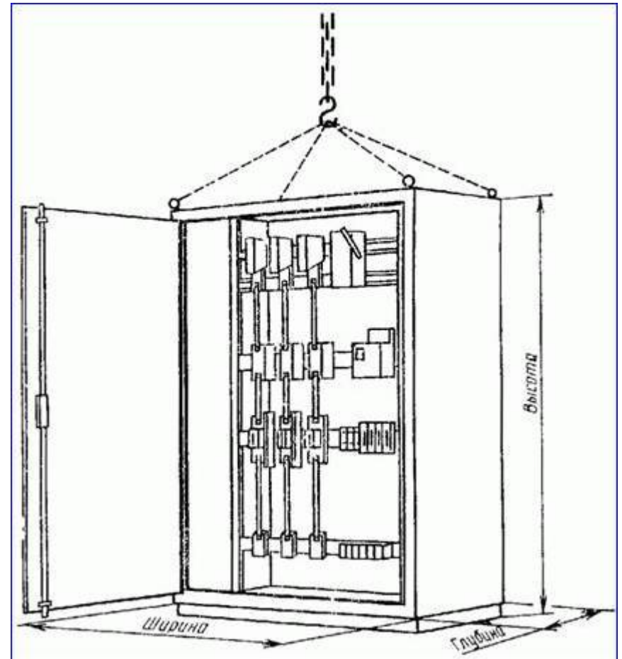
Черт. С3. НКУ заводского изготовления шкафного типа
