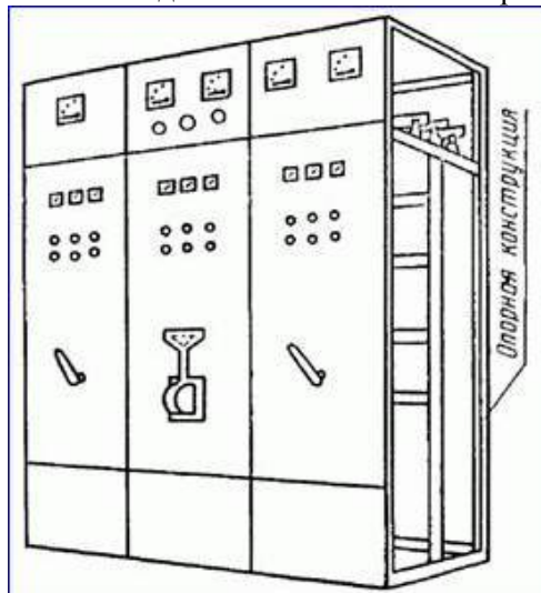
Черт. С2. НКУ заводского изготовления открытого типа, защищенное спереди
