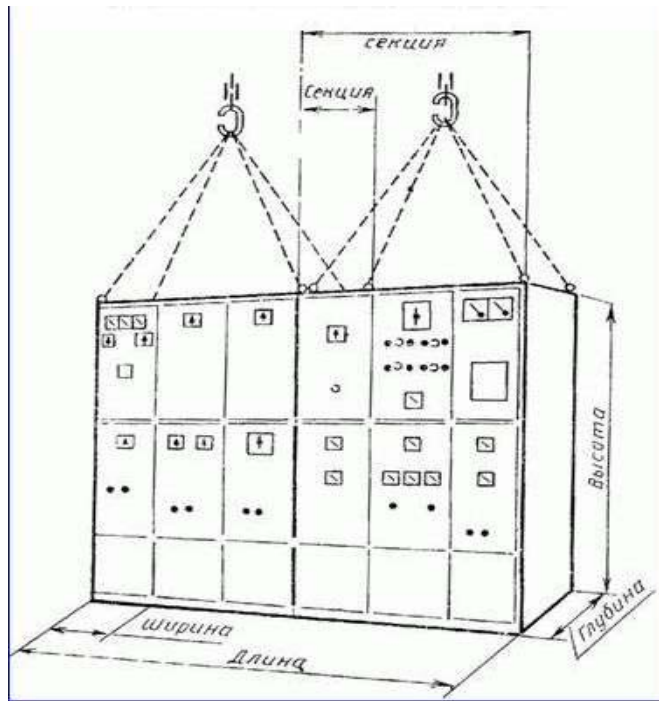
Черт. С4. НКУ заводского изготовления многоящичного типа
