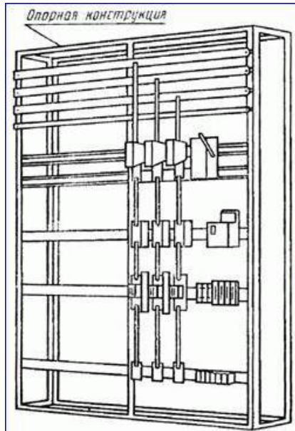
Черт. С1. НКУ заводского изготовления открытого типа
