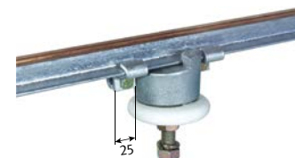
Abbildung zeigt einen Isolator mit 2 Sicherungsklemmen (Festpunkt).
