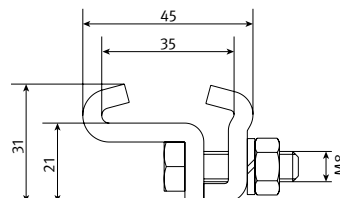
Abbildung zeigt einen Isolator mit 2 Sicherungsklemmen (Festpunkt).
